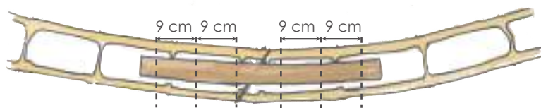
Unión de dos culmos
