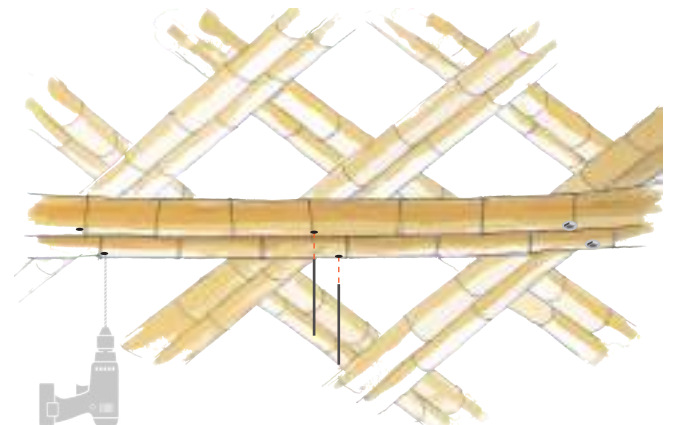
Unión de correa doble a estructura del paraboloides
